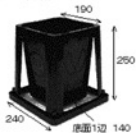
CF-240 (本体)
